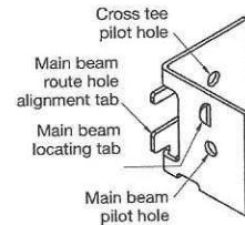
TechZone Bracing Clip (TZBC)
