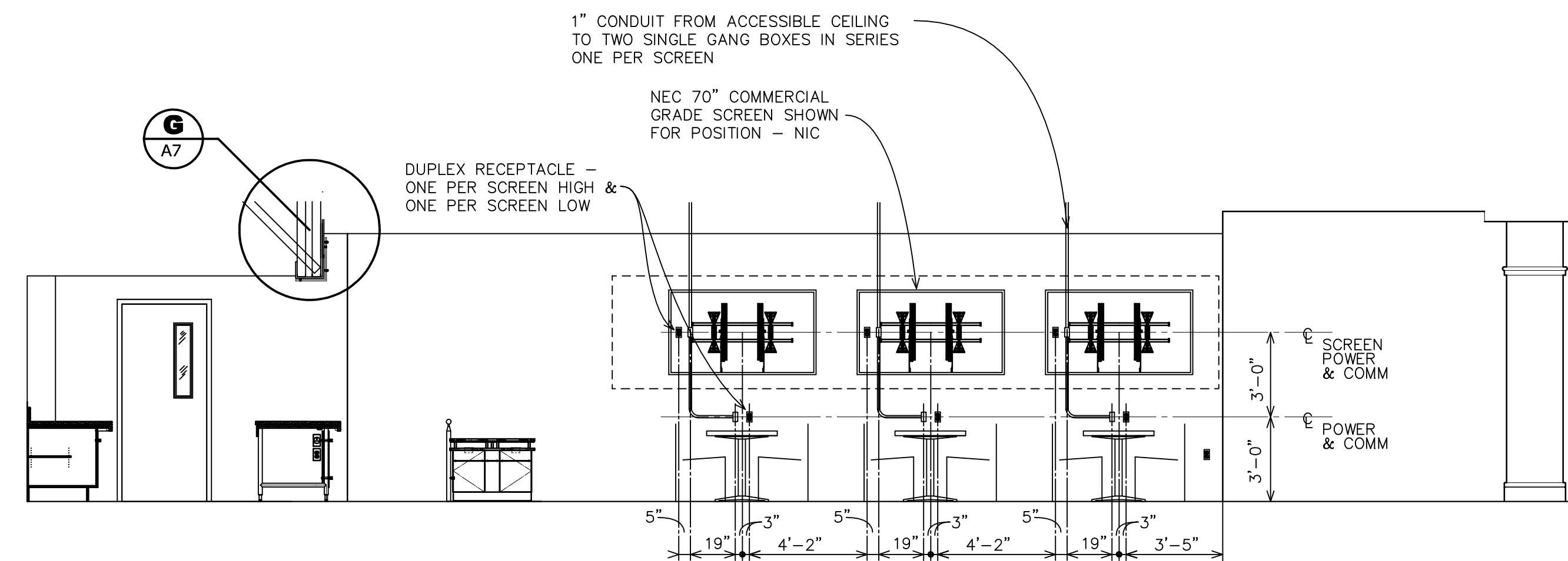
SCALE: 1/4" = 1'-0"
