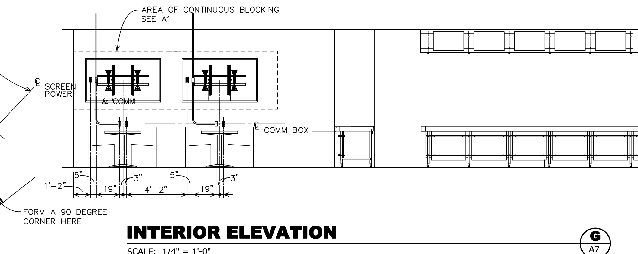
SCALE: 1/4" = 1'-0"
