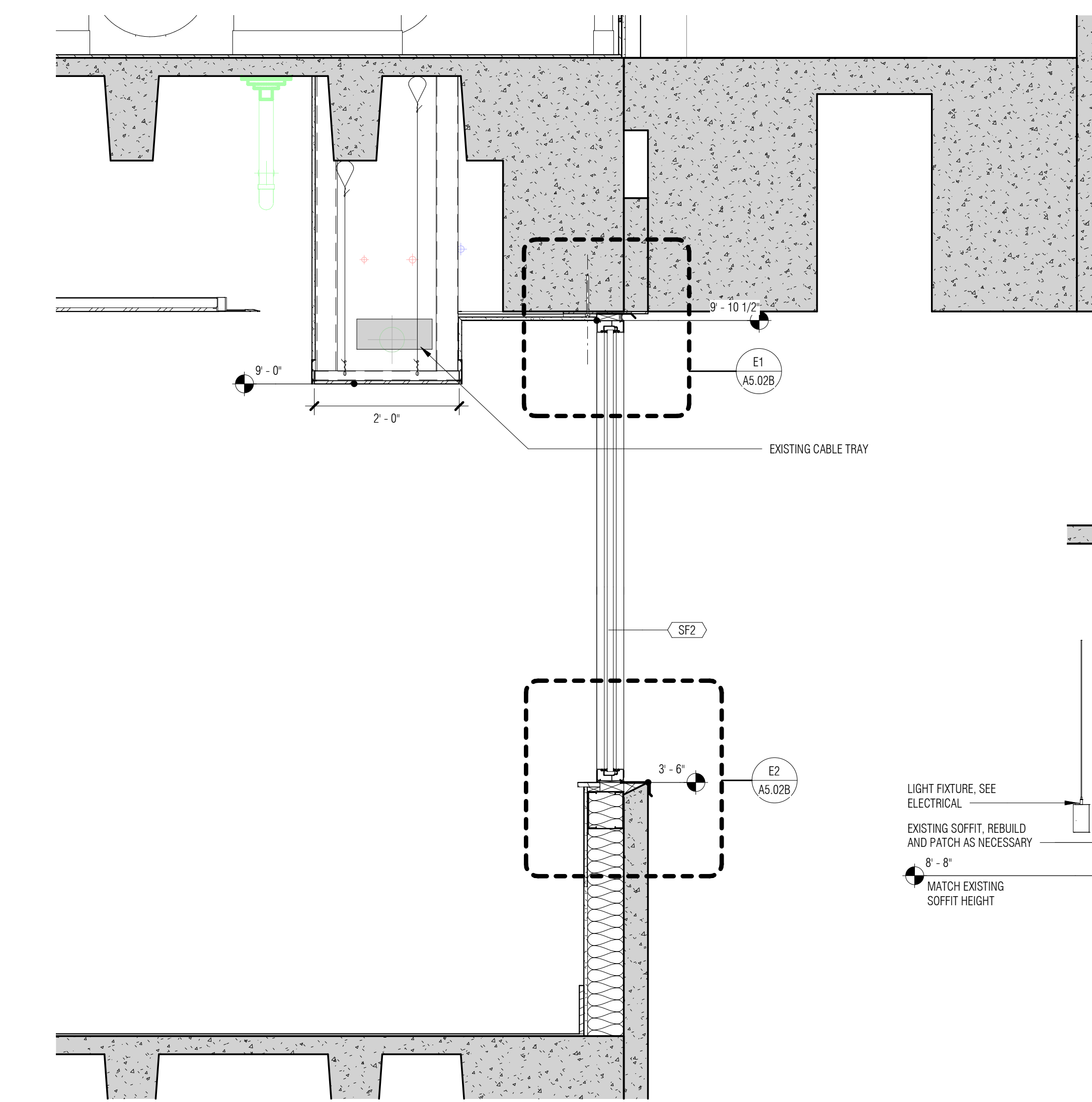
A1 STOREFRONT SECTION A5.02B 3/4" = 1'-0"
