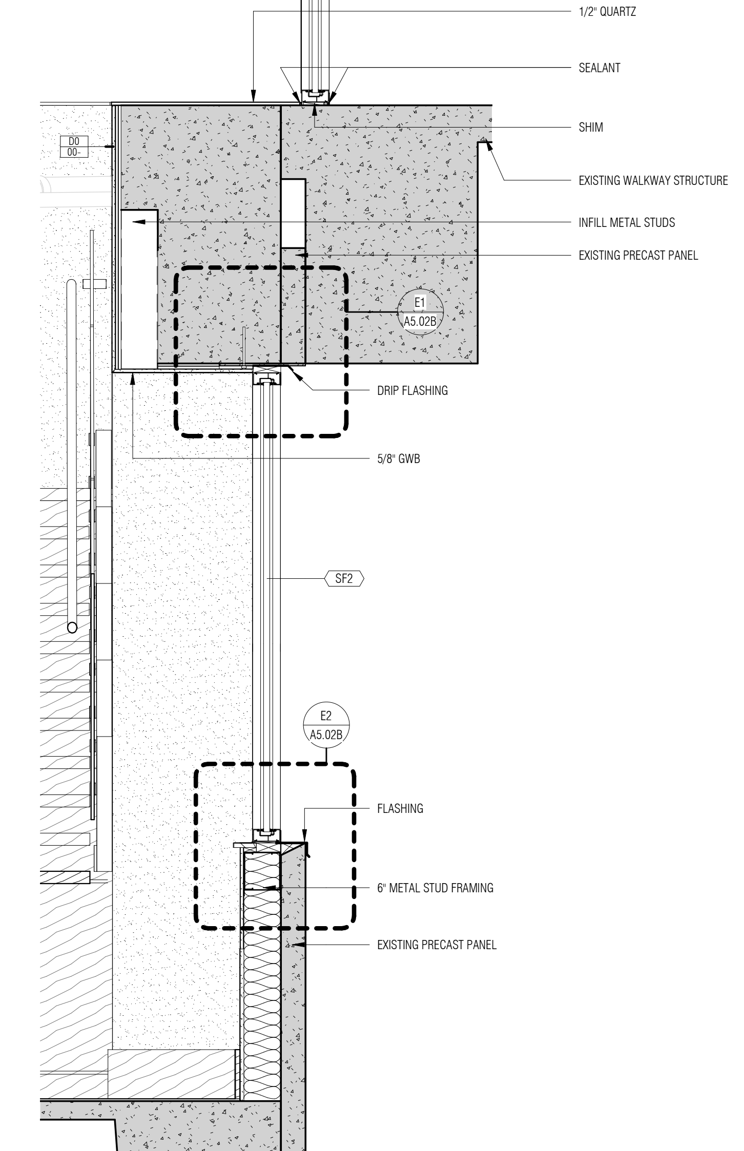
A5 STOREFRONT SECTION A5.02B 3/4" = 1'-0"
