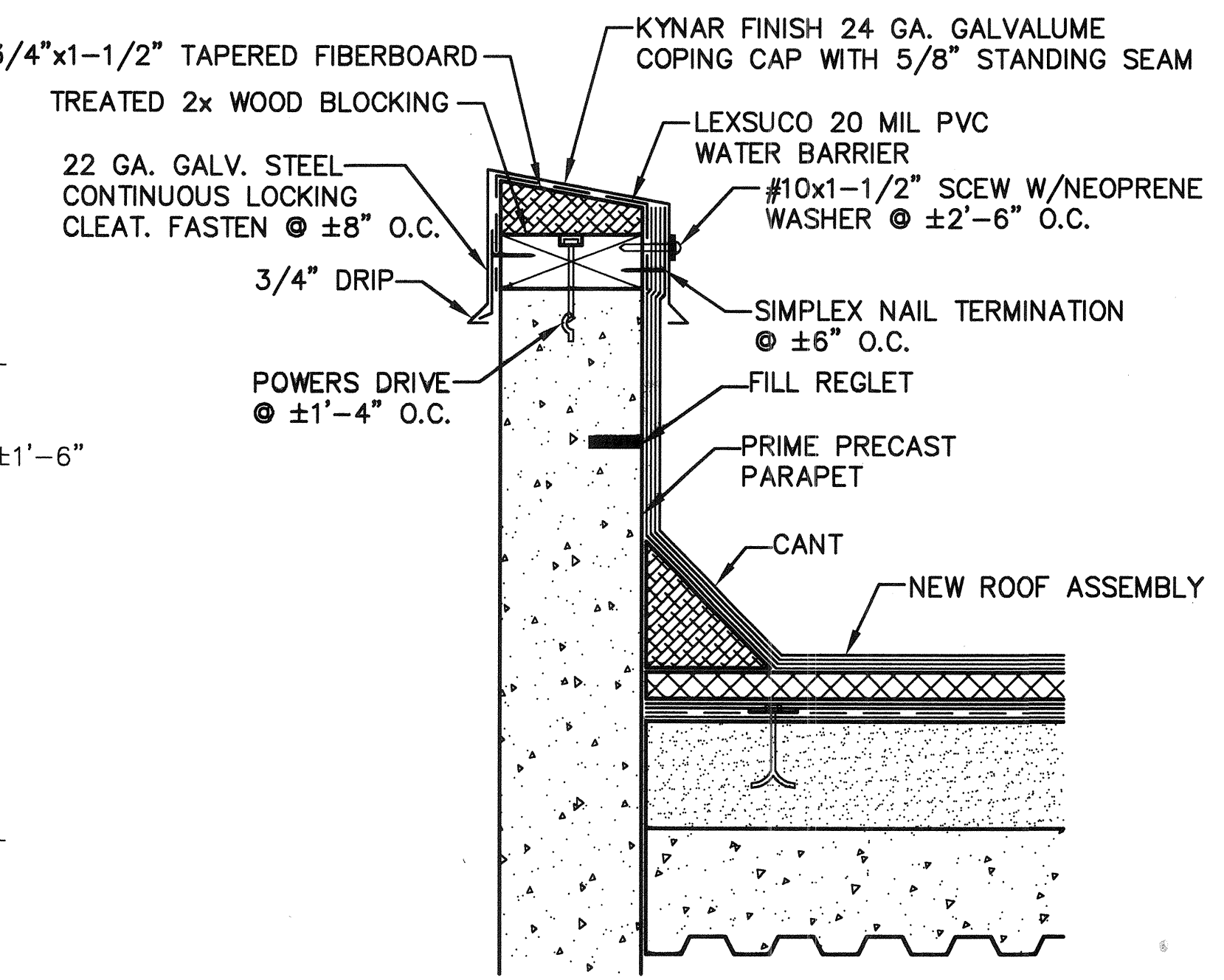
SECTION J-J NTS
